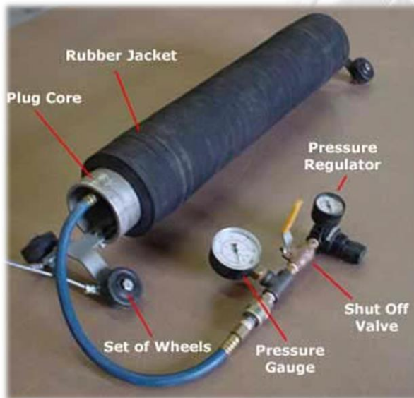
Plugue de instalação
