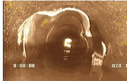
Antes – Vazamento com alta vazão
